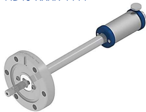
1軸直線回転導入機 MD40-XXXX-YYYY
