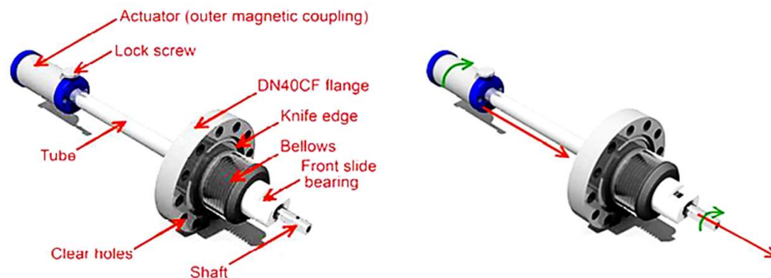
【1軸ウォブルスティック各部名称とハンドリング】 WM40-XXXX-YYYY
