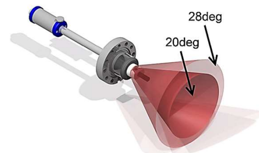
【振れ角】 WM40: \pm 20^\circ WMWA40: \pm 20^\circ
