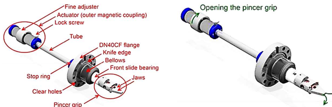
【WMG40(FC)-PGWMS(OM) 高精度2軸ICF70ウォブルスティック各部名称とハンドリング】
