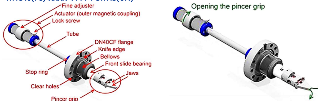
【高精度2軸ウォブルスティック各部名称とハンドリング】 WMG40(FC)-XXXX-YYYY-PGWMS(OM)
