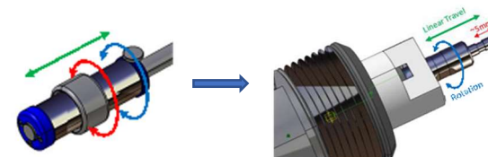
WMG40(FC) : 動作図
