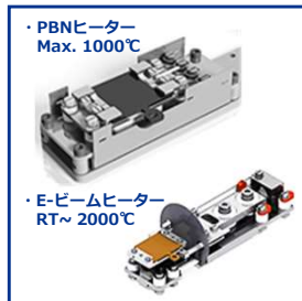
サンプルプレートヒーター
