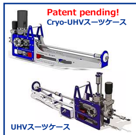
UHVスーツケース
