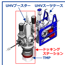
高速真空排気ドッキングステーション
