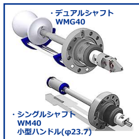
ウォブルスティック
