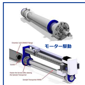
サンプルトランスポーター
