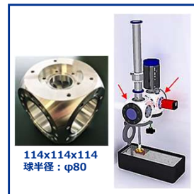
高強度Al合金製球形キューブ
