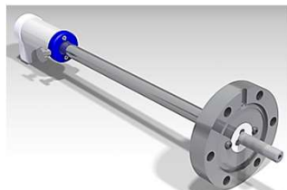
MD40(RL) アングルリミッター 直線回転導入機
