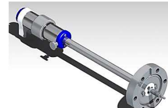
MDG40(RL) アングルリミッター デュアルシャフト直線回転導入機
